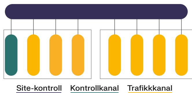
Figur 4. Basestasjon med to baseradioer.
