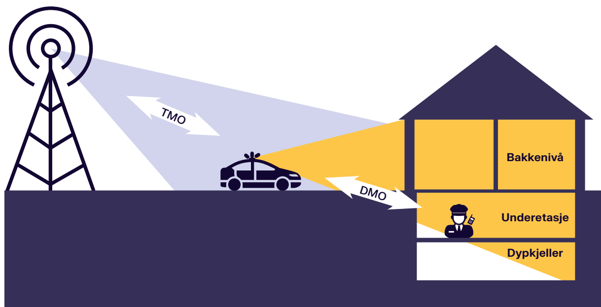
Figur 6. Eksempel på Gateway plassert i bil for å binde brukere i TMO og DMO sammen.
