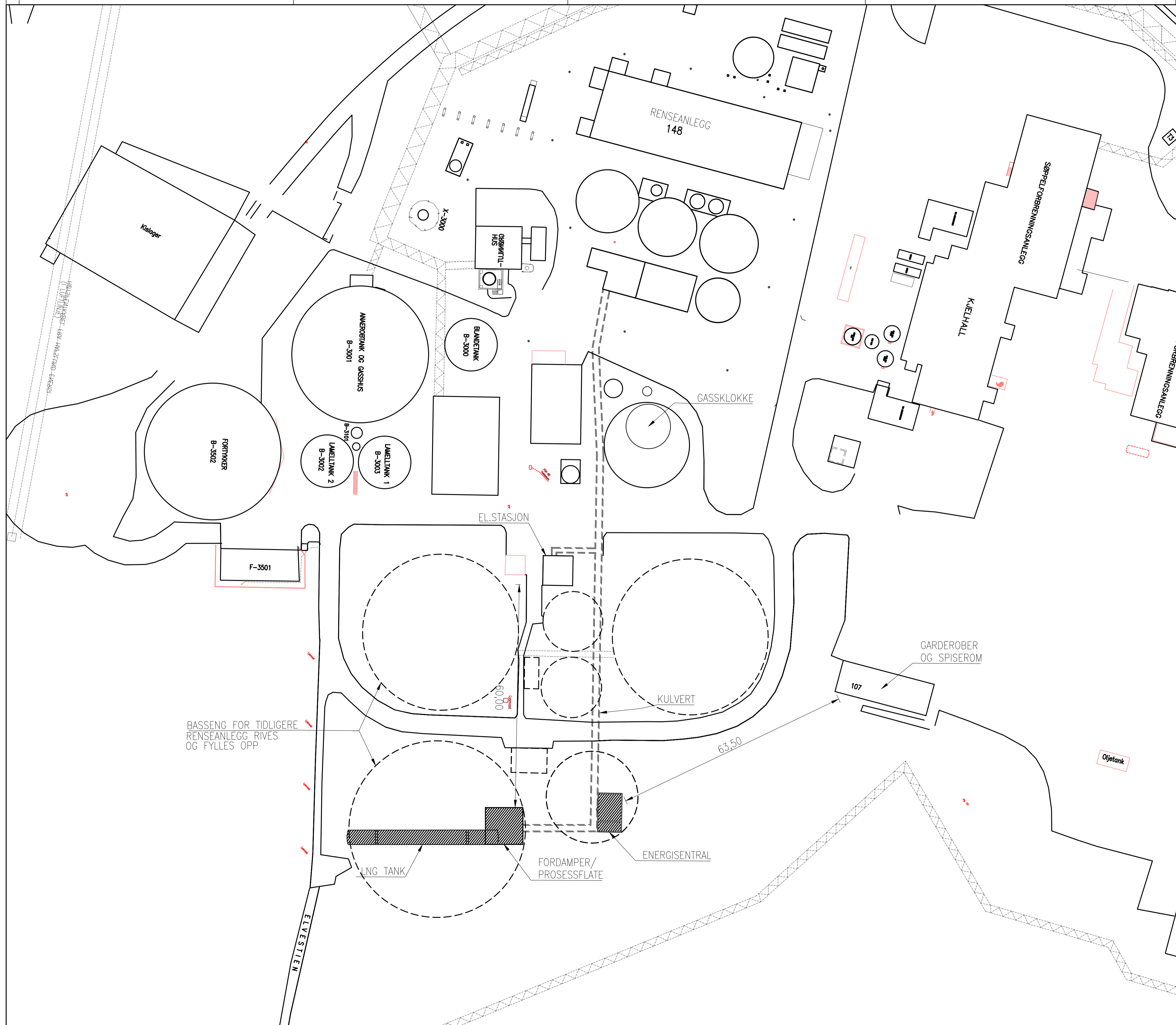
SITUASJONSPLAN 1:500
